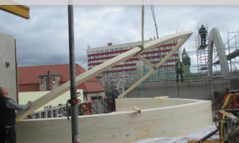
ZOLLINGERDACH in Einzelteilen
